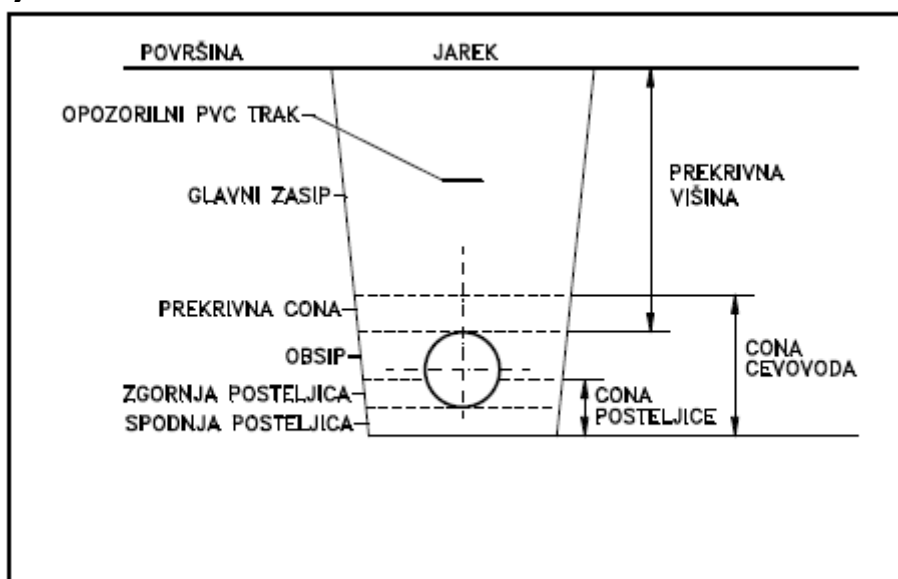
Slika 1: Prerez jarka
